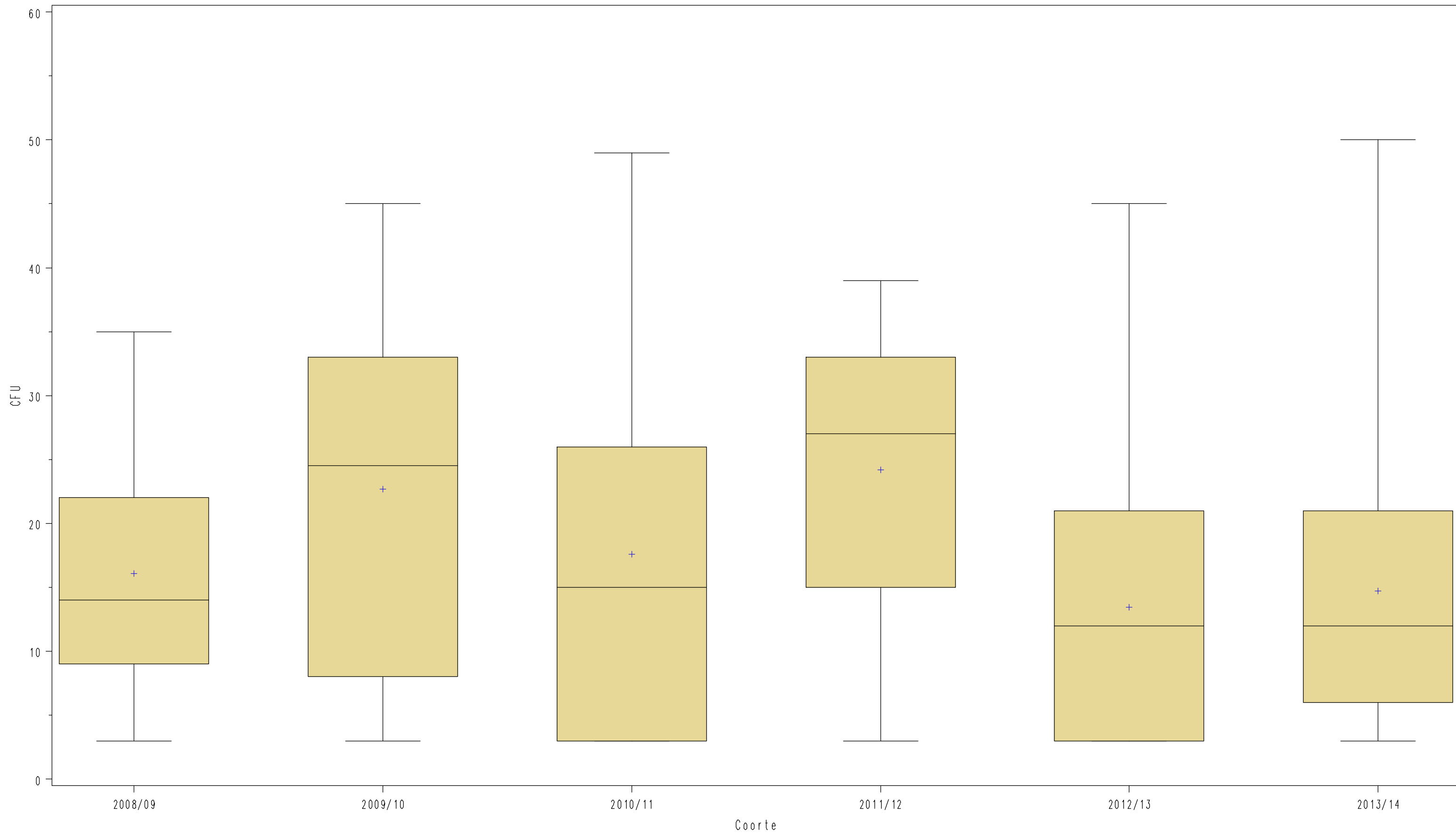
FIGURA 1.4 L - BOX-PLOT DEI CFU ACQUISITI DAGLI STUDENTI AL 31/07 DEL I ANNO
