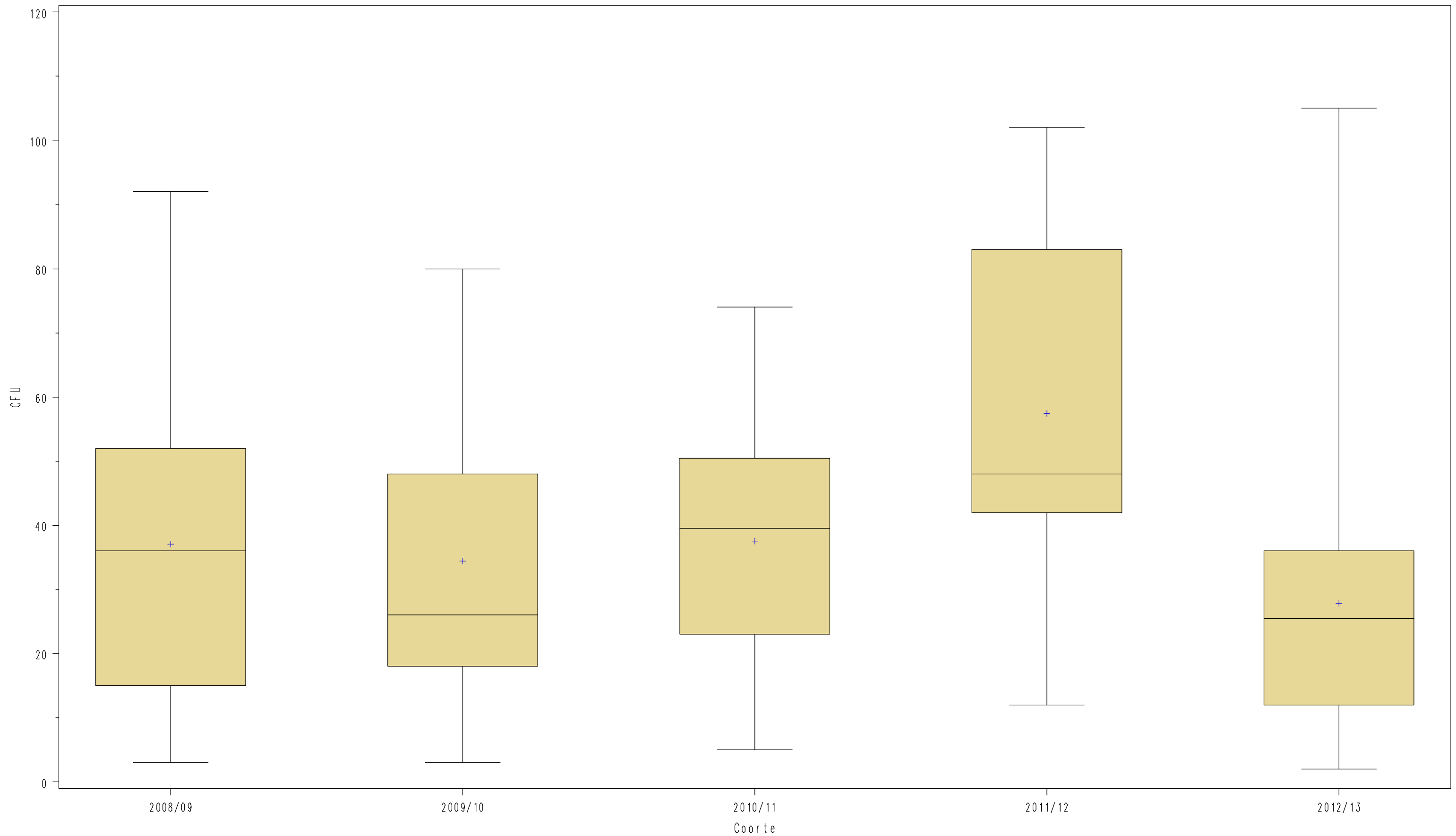
FIGURA 1.5 L - BOX-PLOT DEI CFU ACQUISITI DALLE COORTI AL 31/07 DEL II ANNO
